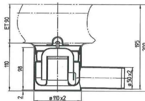
vue du raccord
