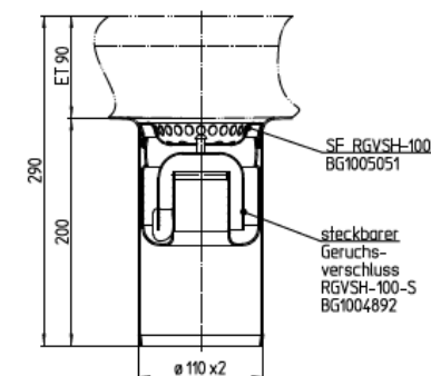
vue du raccord
