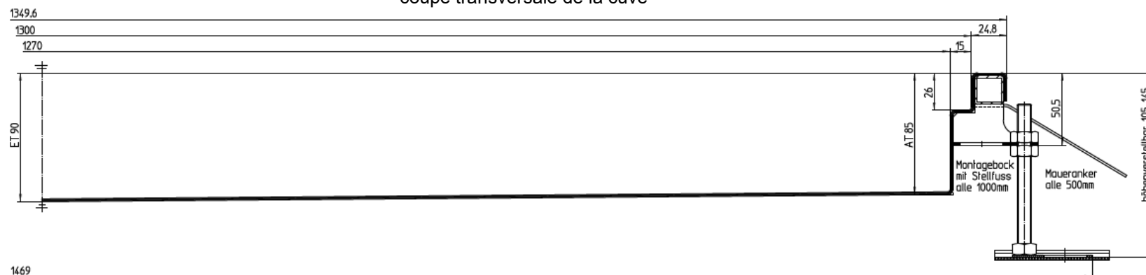
coupe transversale de la cuve
