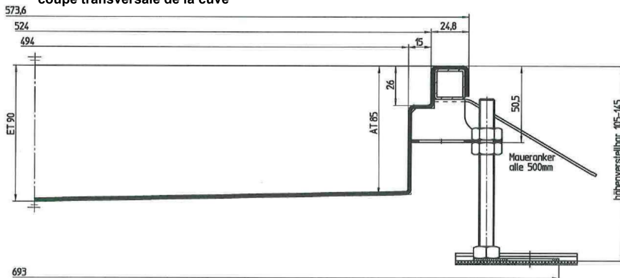
coupe transversale de la cuve
