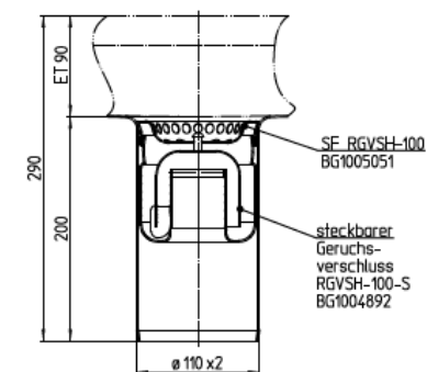
Stützen-Ansicht
