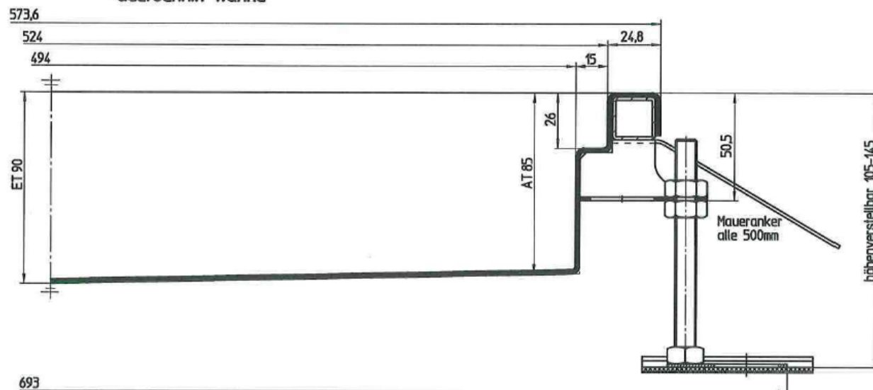
Querschnitt Wanne
