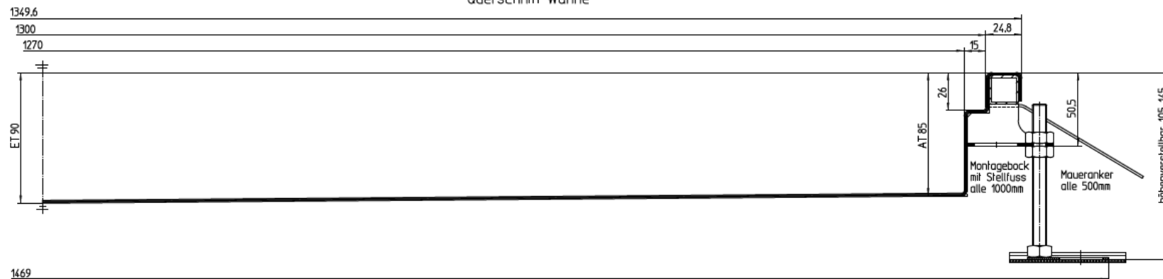
Querschnitt Wanne
