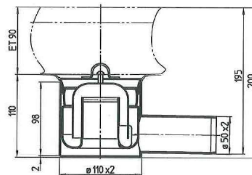
Stützen-Ansicht
